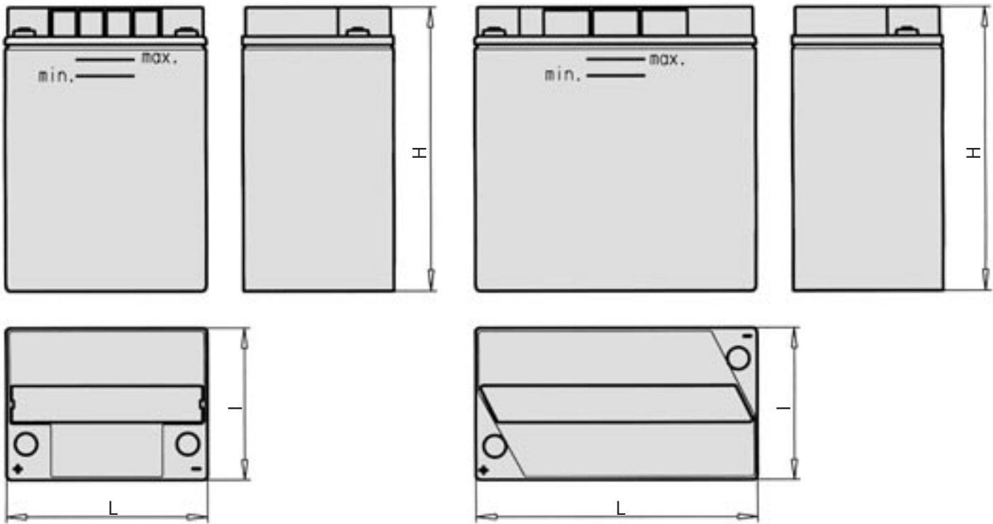
12 V 1 OPzS 50 - 12 V 3 OPzS 150
